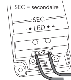
b. effectuez les connexions entre le transfo et le ou les luminaires
